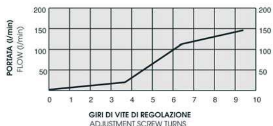
GRAFICO PORTATE PER SILENZIATORI REGOLATI 1/4" A 0,254 bar TYPICAL FLOW TEST GRAPH FOR 1/4" RESTRICTOR 0.254 bar
